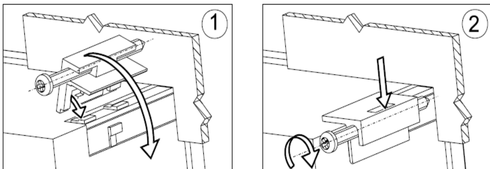
Рис. 1. Монтаж прибора на щит
