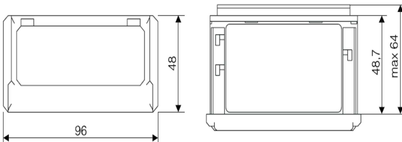
Рис. 2. Габариты прибора
