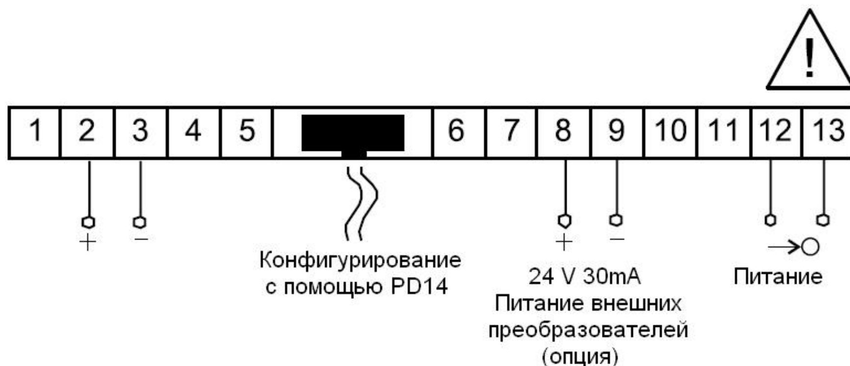
Рис. 3. Схема электрических соединений для приборов N24S и N25S
